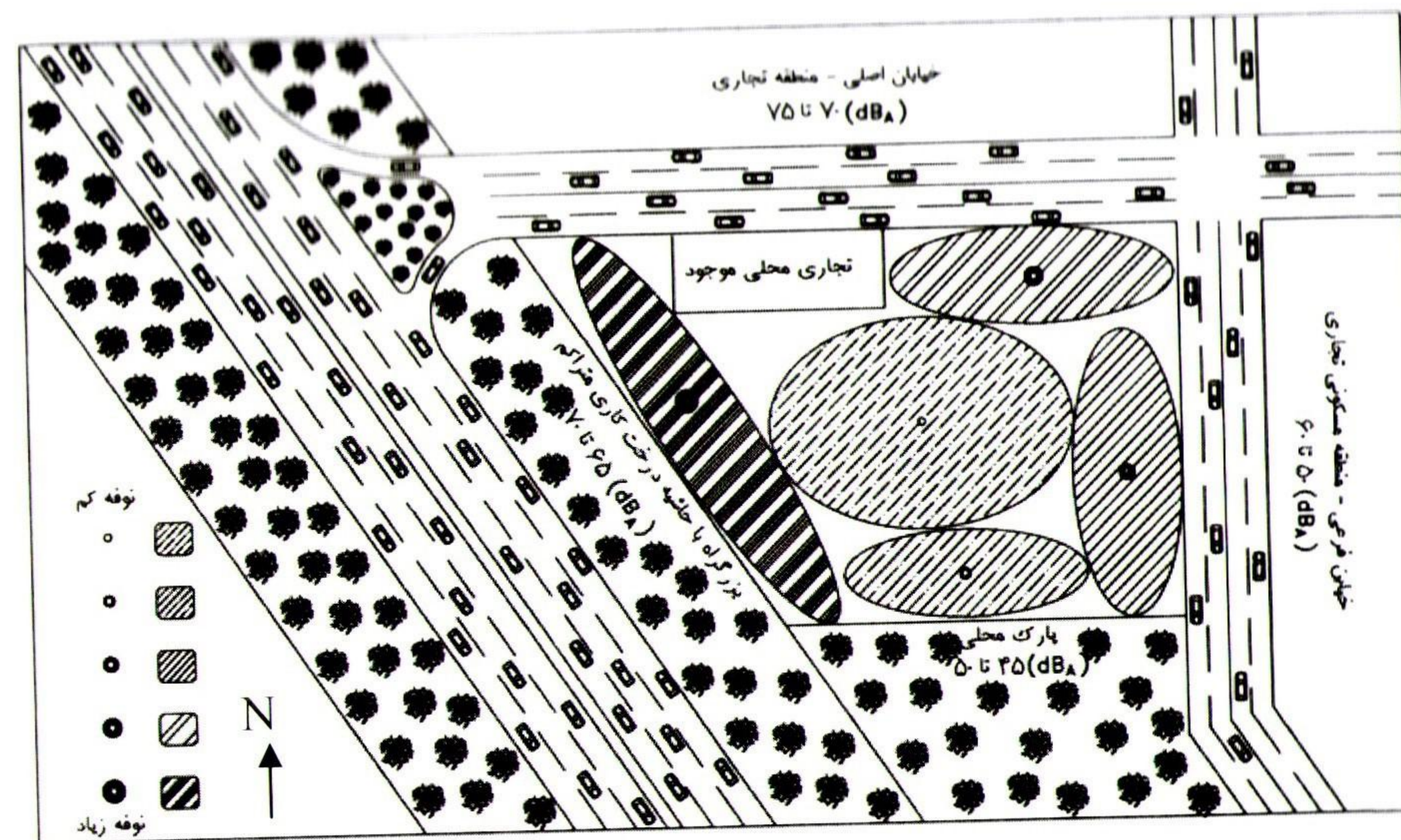
شکل پ ۵-۶: منطقه‌بندی از نظر آکوستیکی در سایت فرضی
