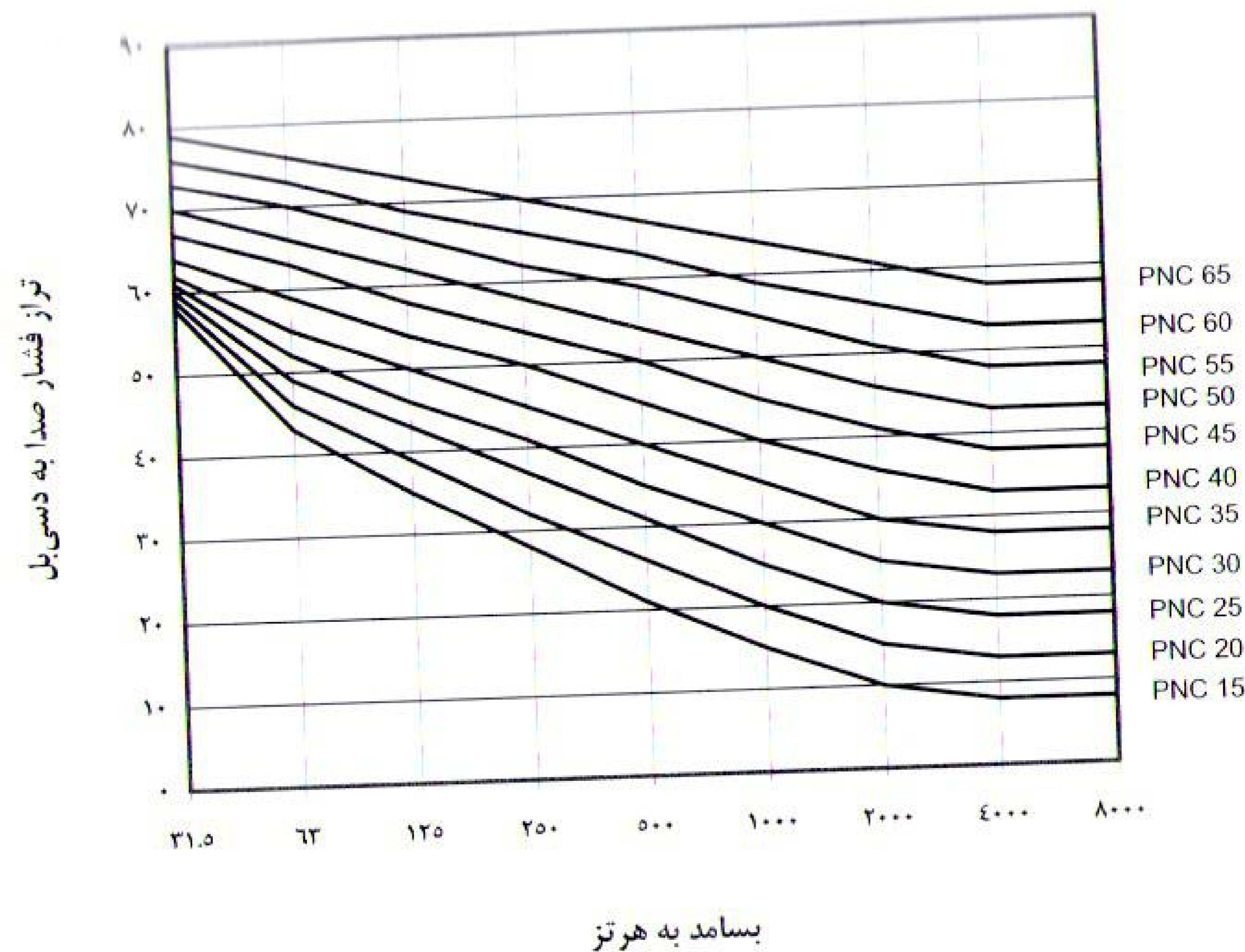
شکل ۱-۱۸-۳-۵: نمودارهای برسنج ترجیحی نوفه PNC
