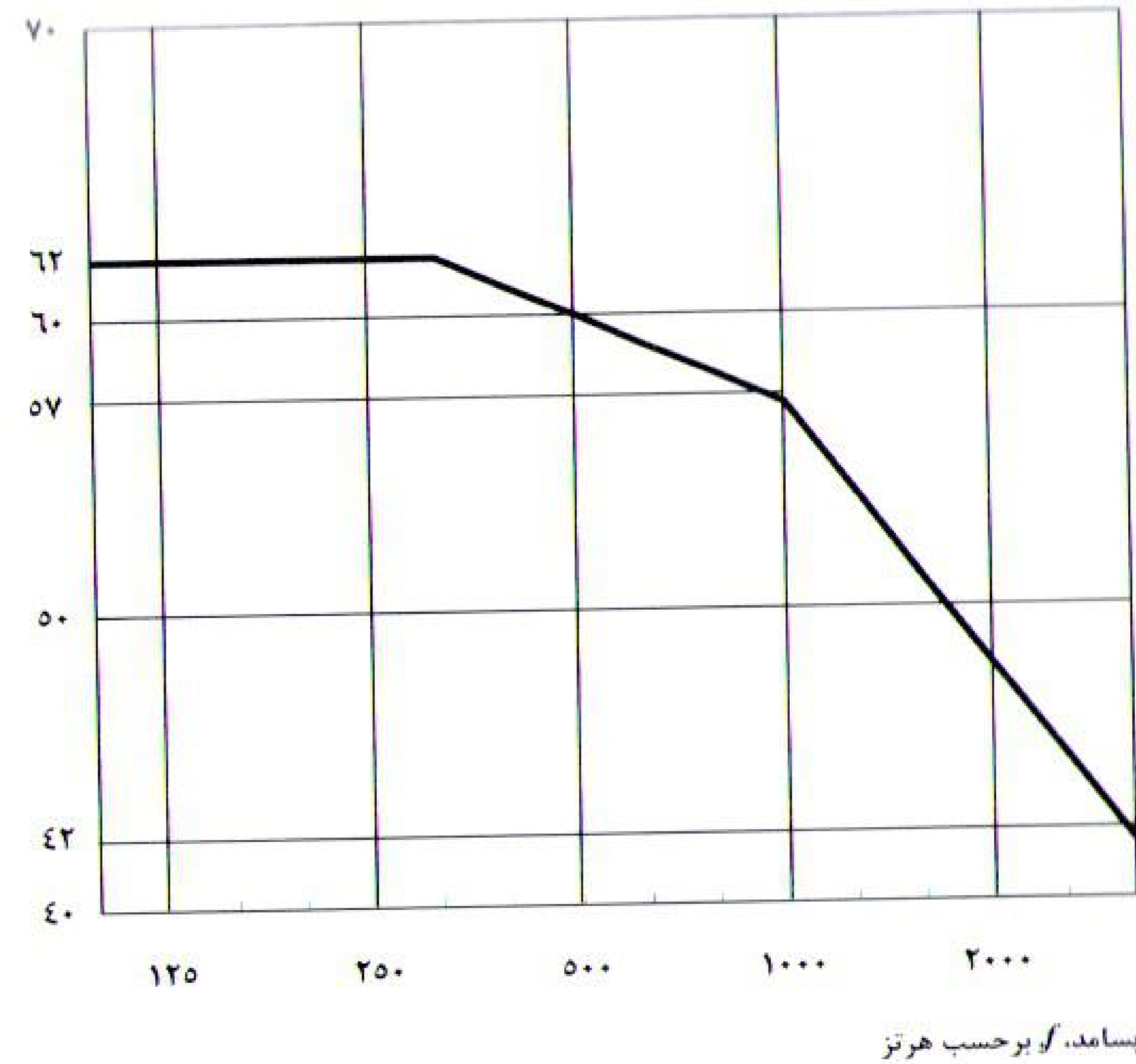
شکل ۱-۱۸-۳-۱: نمودار مقادیر مینا برای صدای کوبه‌ای، در بندهای یک‌سوم هنگامی
