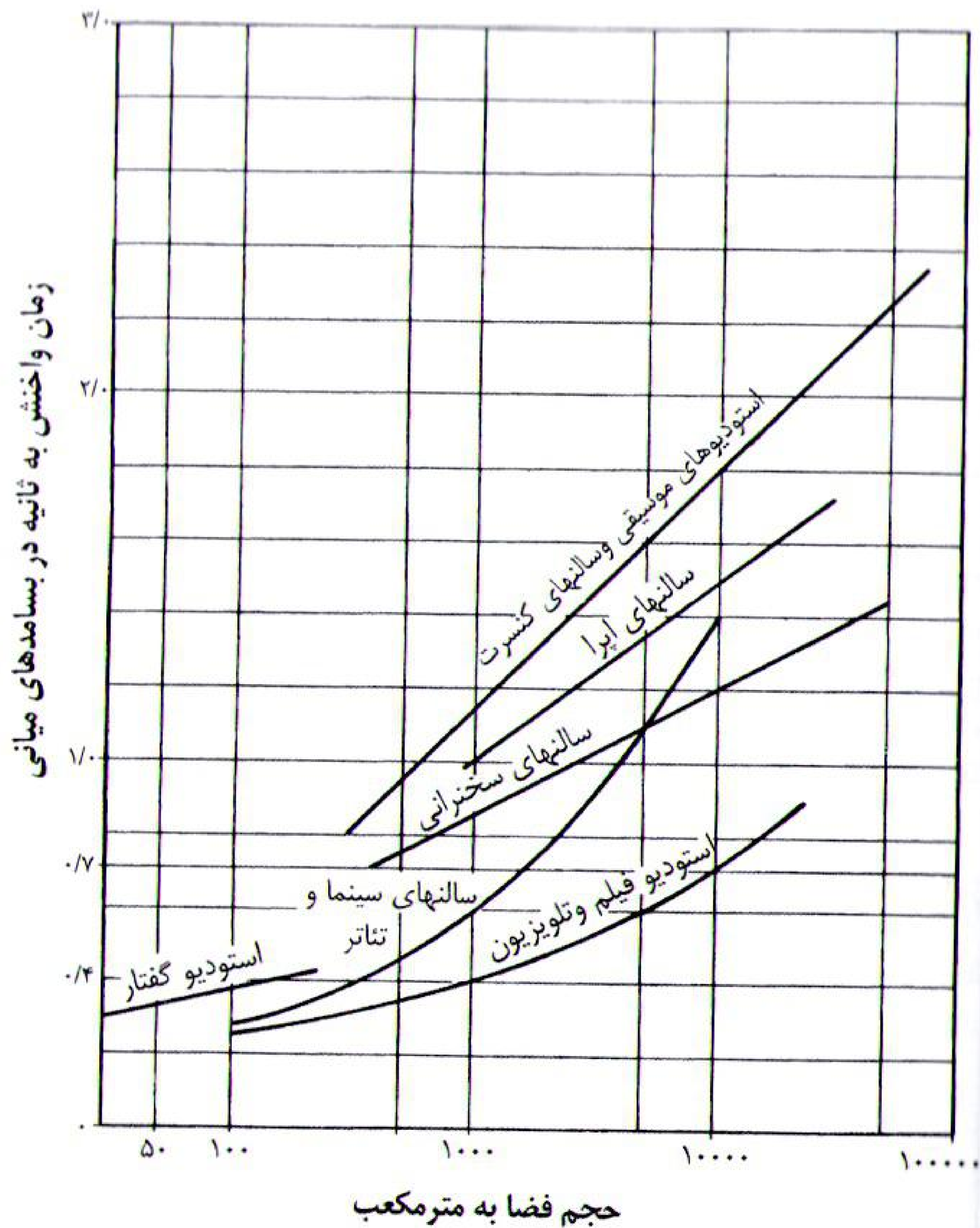
شکل ۱۸-۲-۷-۱: نمودار زمان واخنش بهینه در فضاهای مختلف
