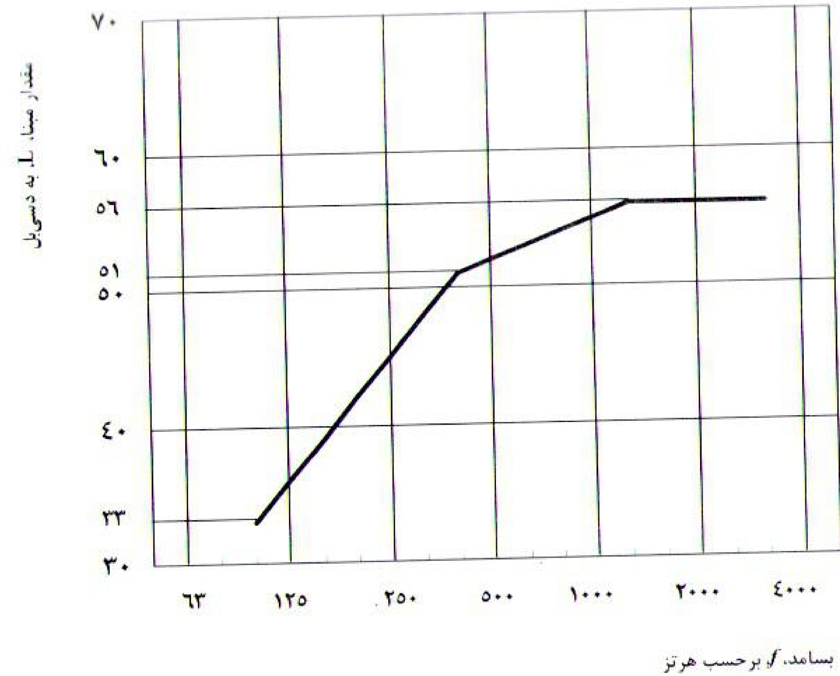
شکل ۱-۱۸-۳-۴: نمودار مقادیر مینا برای صدای هوابرد، در بندهای یک‌سوم هنگامی
